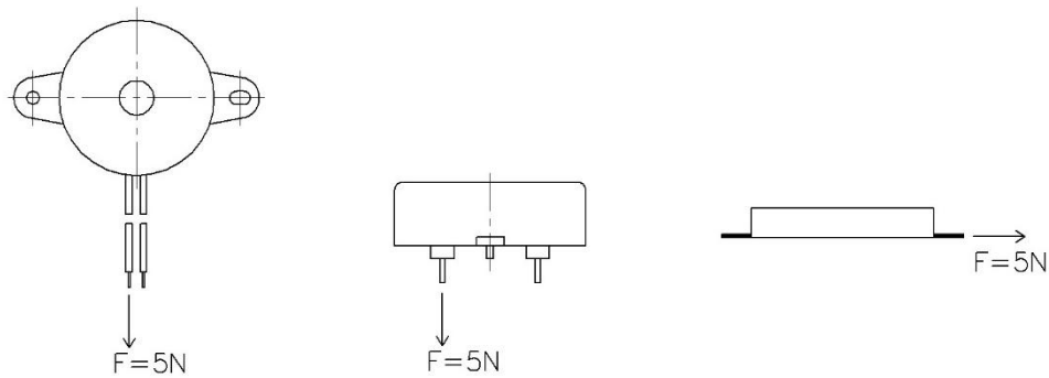
图 6 拉力强度试验示意图
